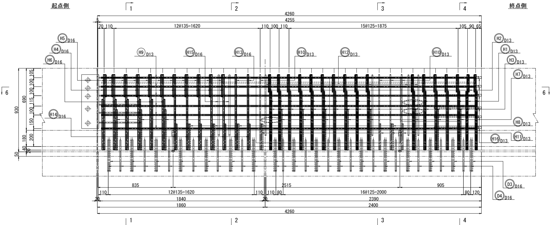
平面図
