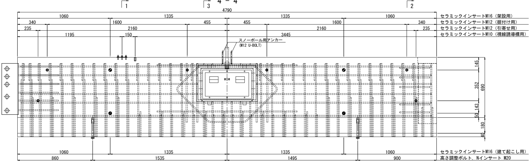
インサート配置側面図
