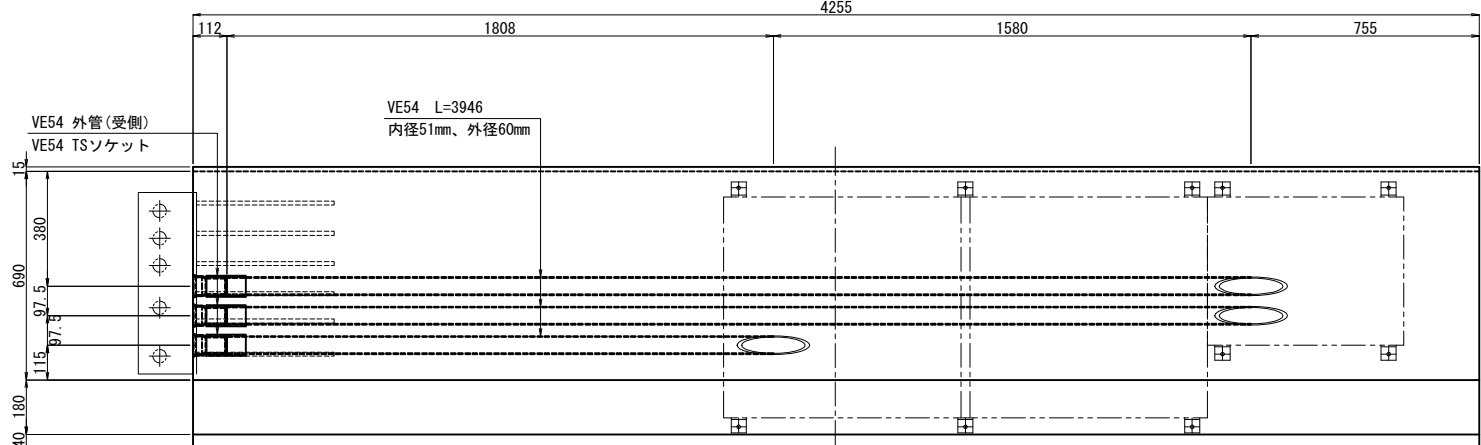
埋設管配置側面図
