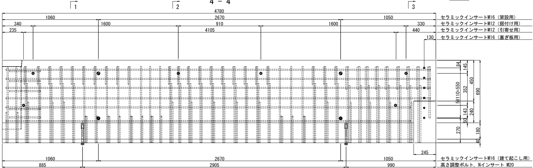
インサート配置側面図
