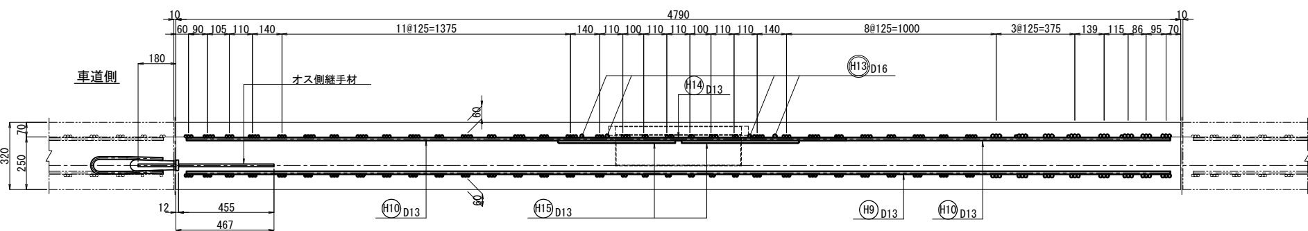
平面図
