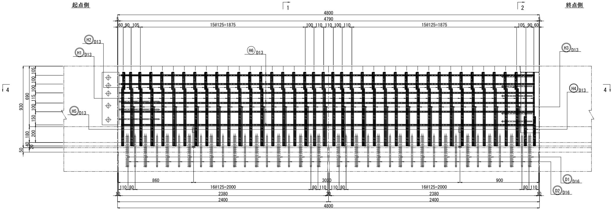
側面図 3 - 3
