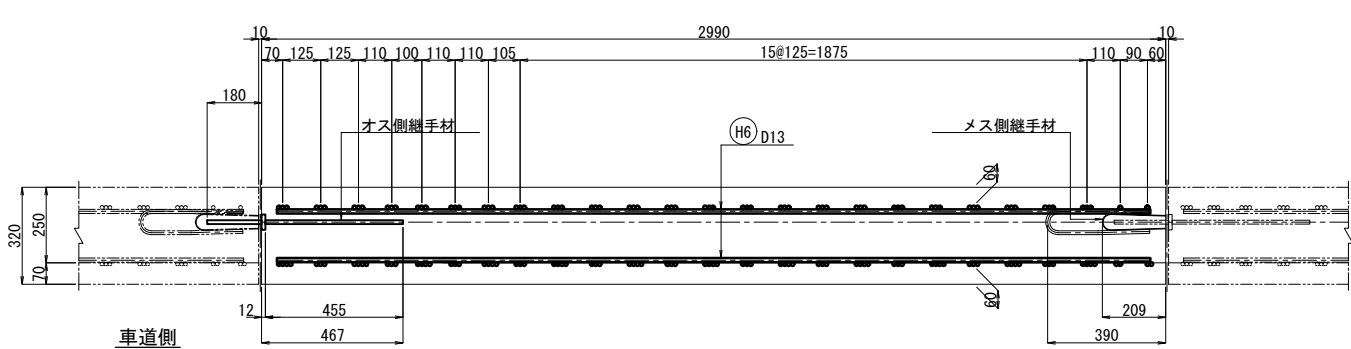
平面図
