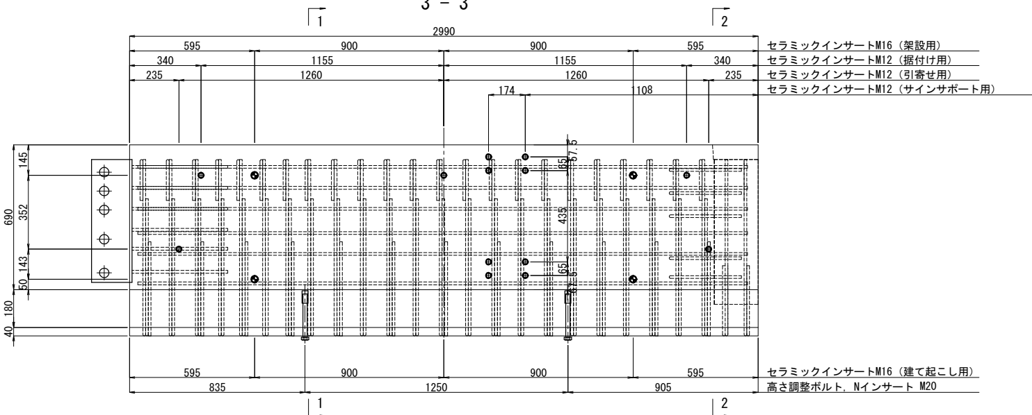
インサート配置側面図
