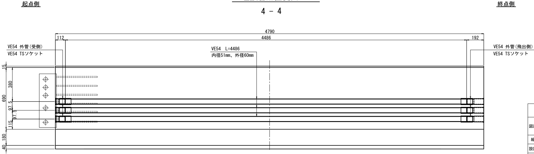
埋設管配置側面図
