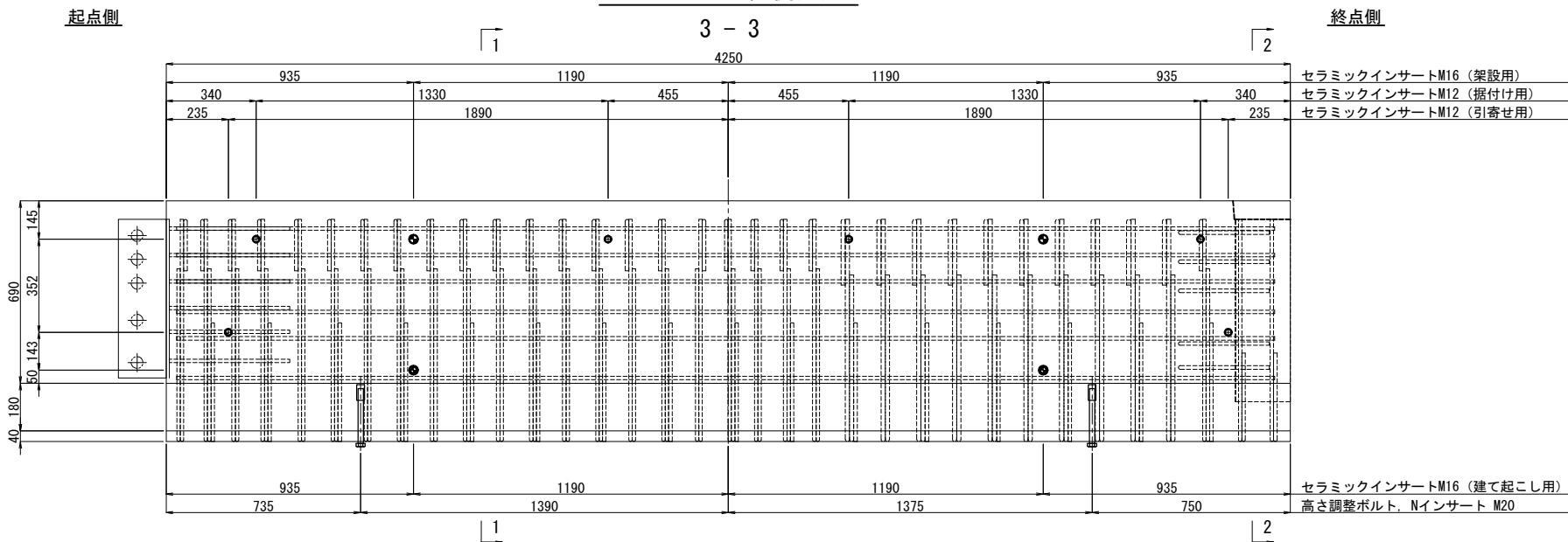
インサート配置側面図
