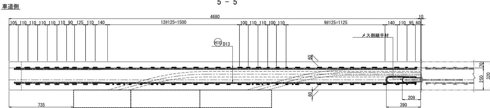
平面図
