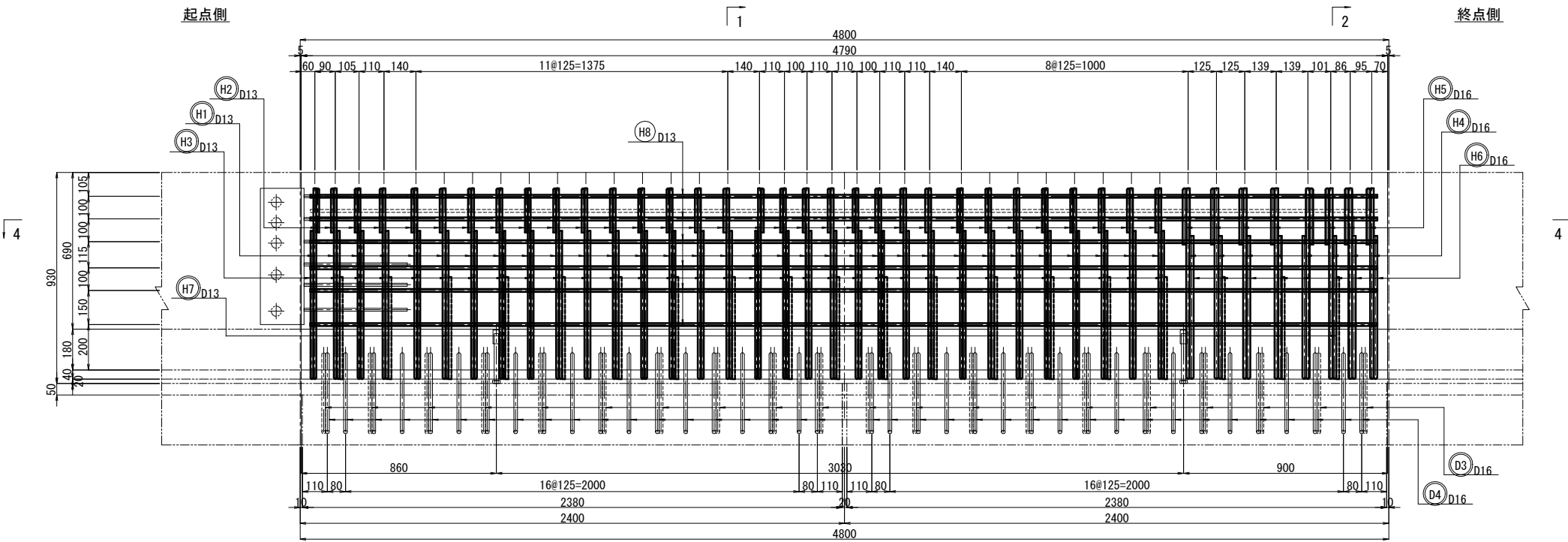
側面図
