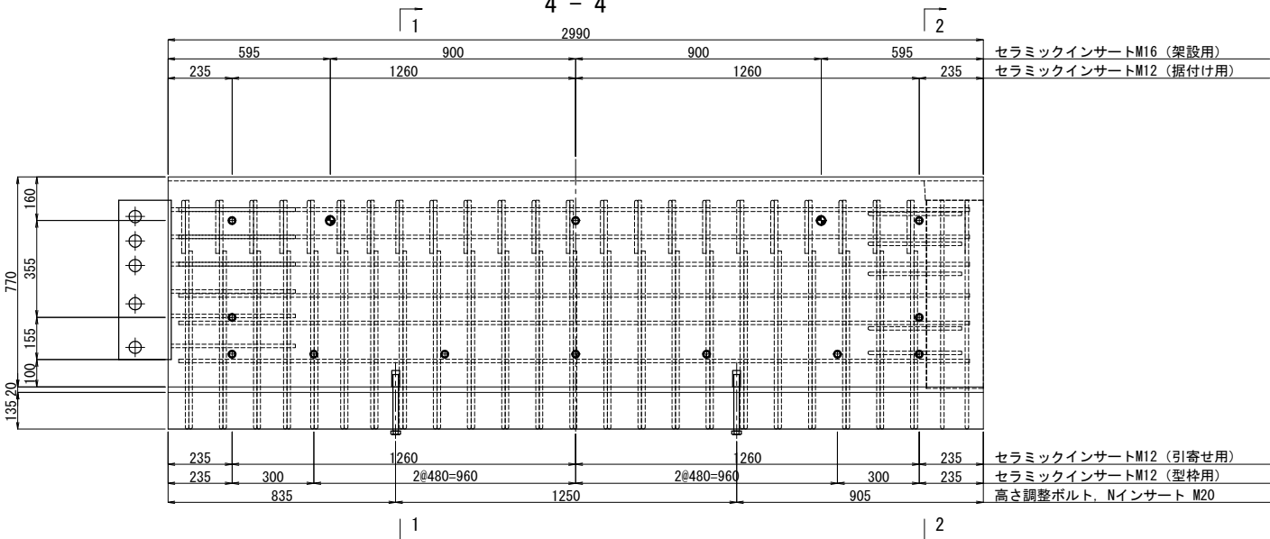
埋設管配置側面図
