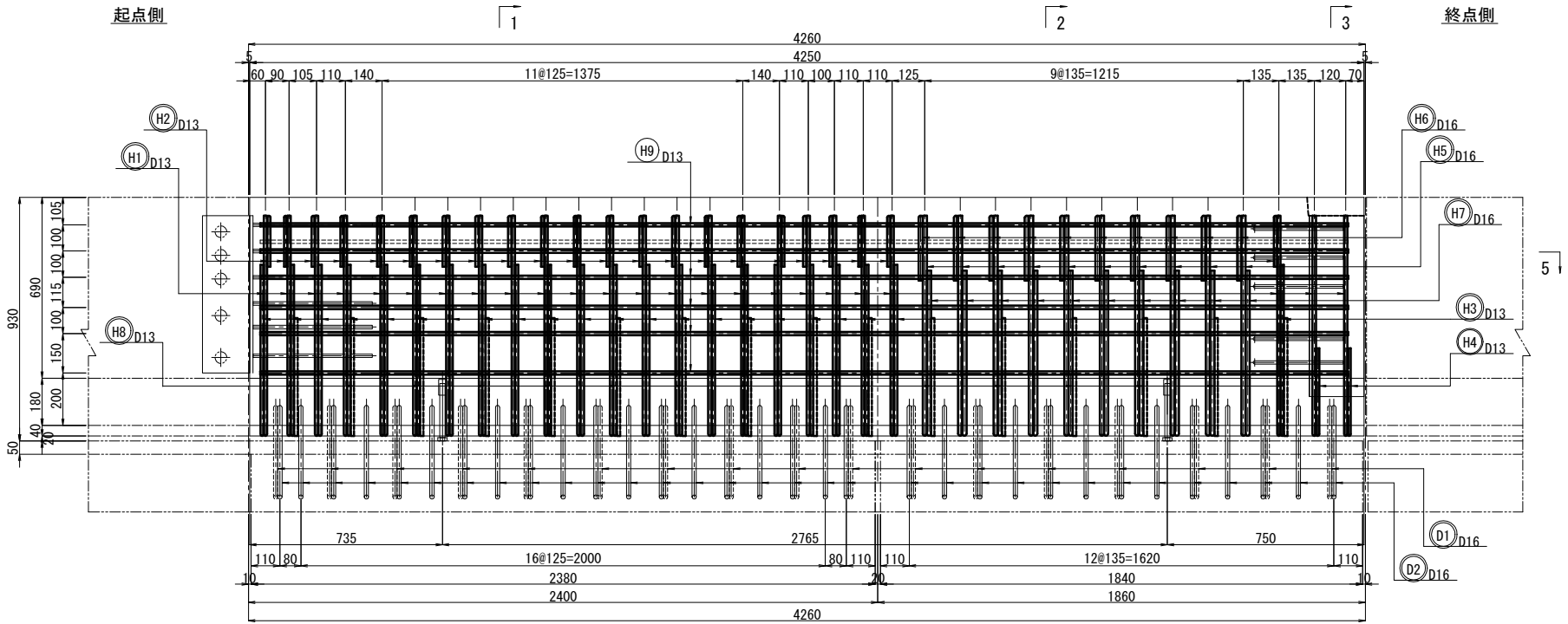
側面図
