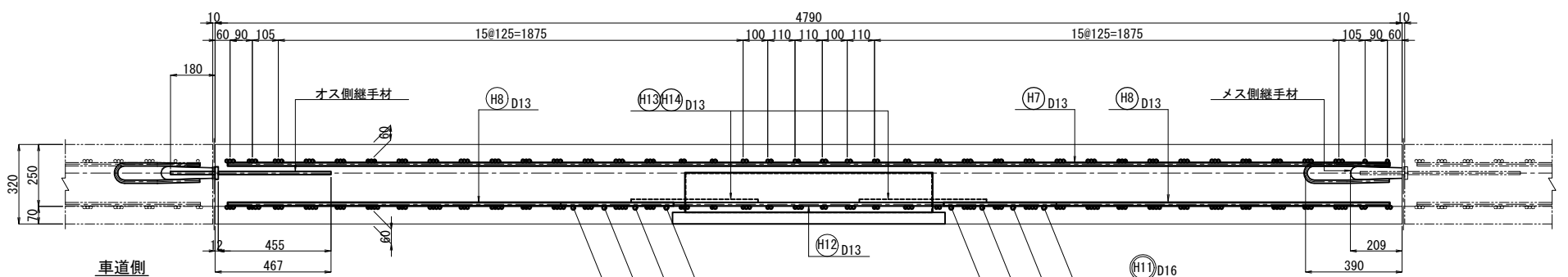
平面图 5 - 5
