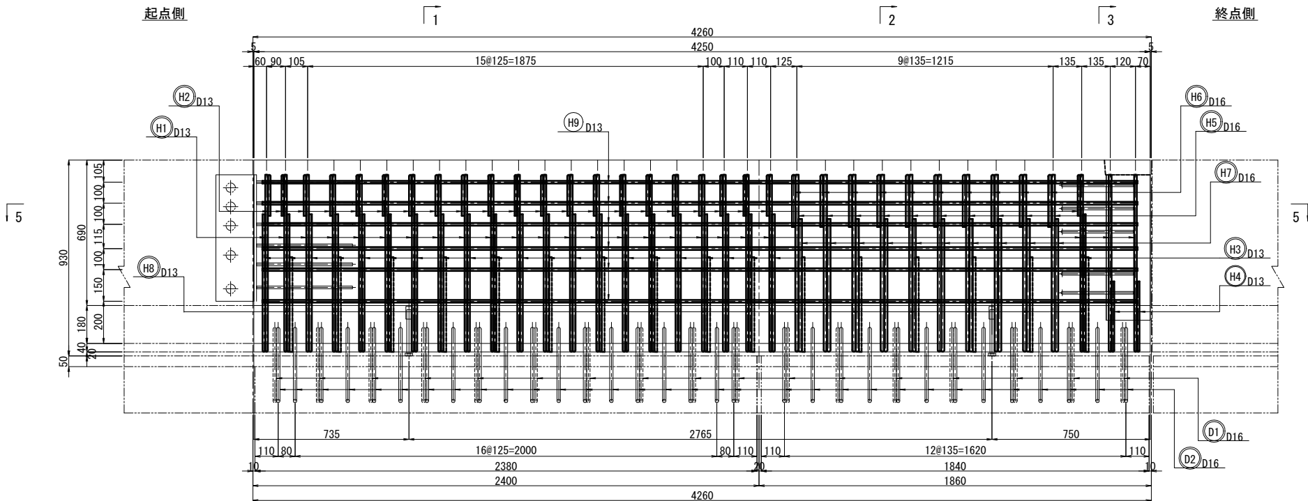
側面図 4 - 4
