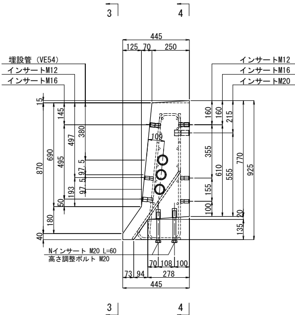
断面図 1 - 1
