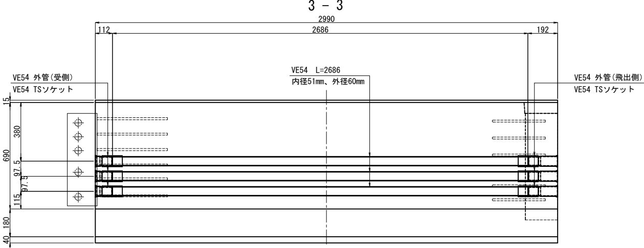
埋設管配置側面図
