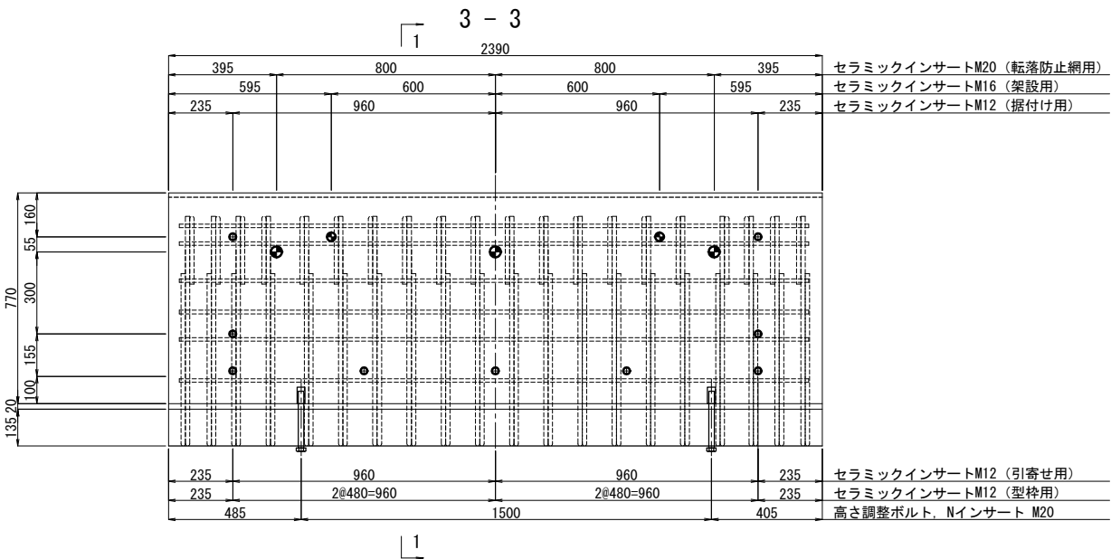
埋設管配置側面図
