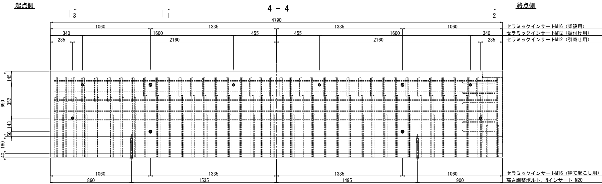
インサート配置側面図
