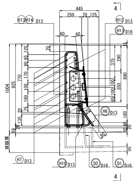
断面図 3 - 3
