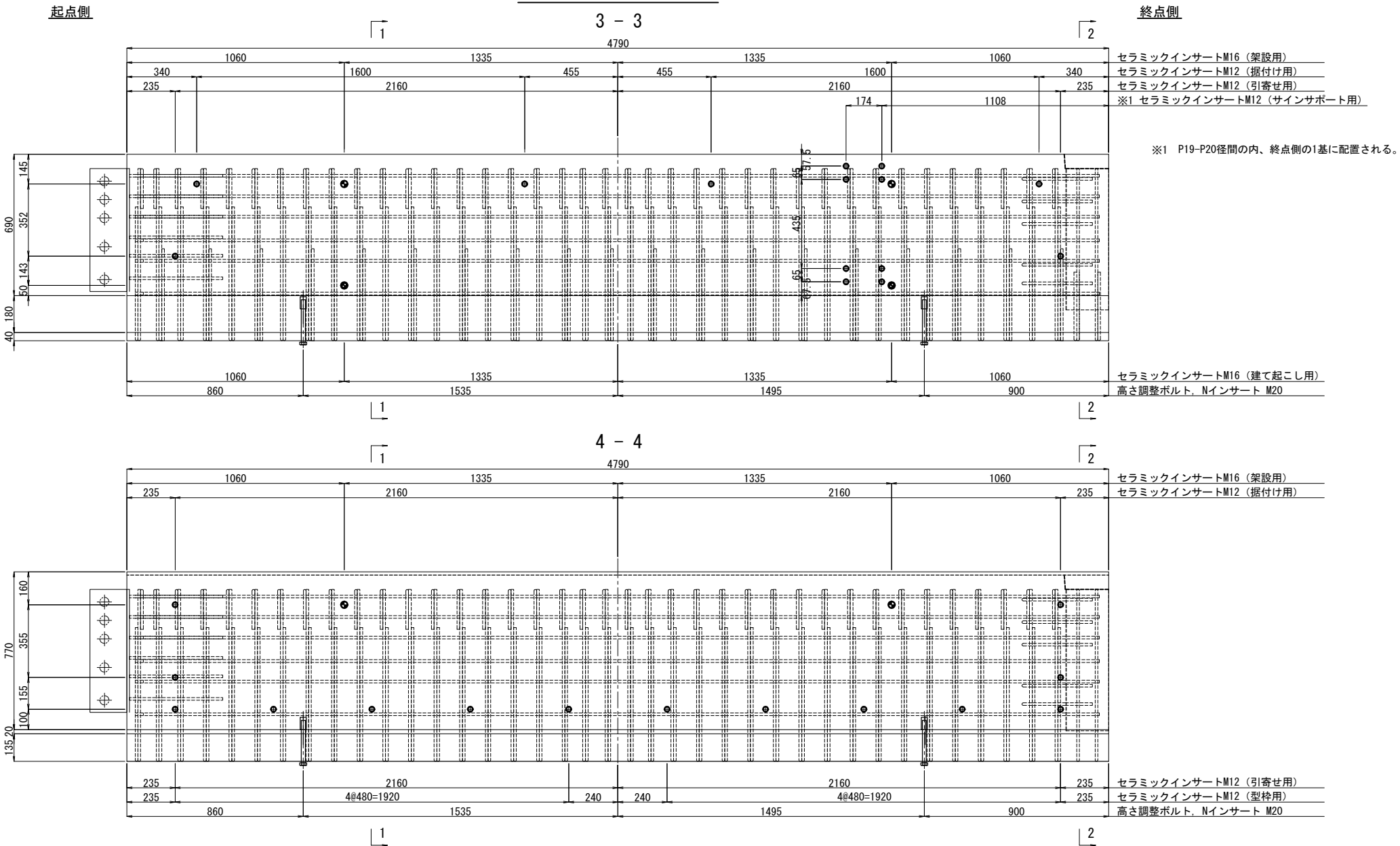
埋設管配置側面図
