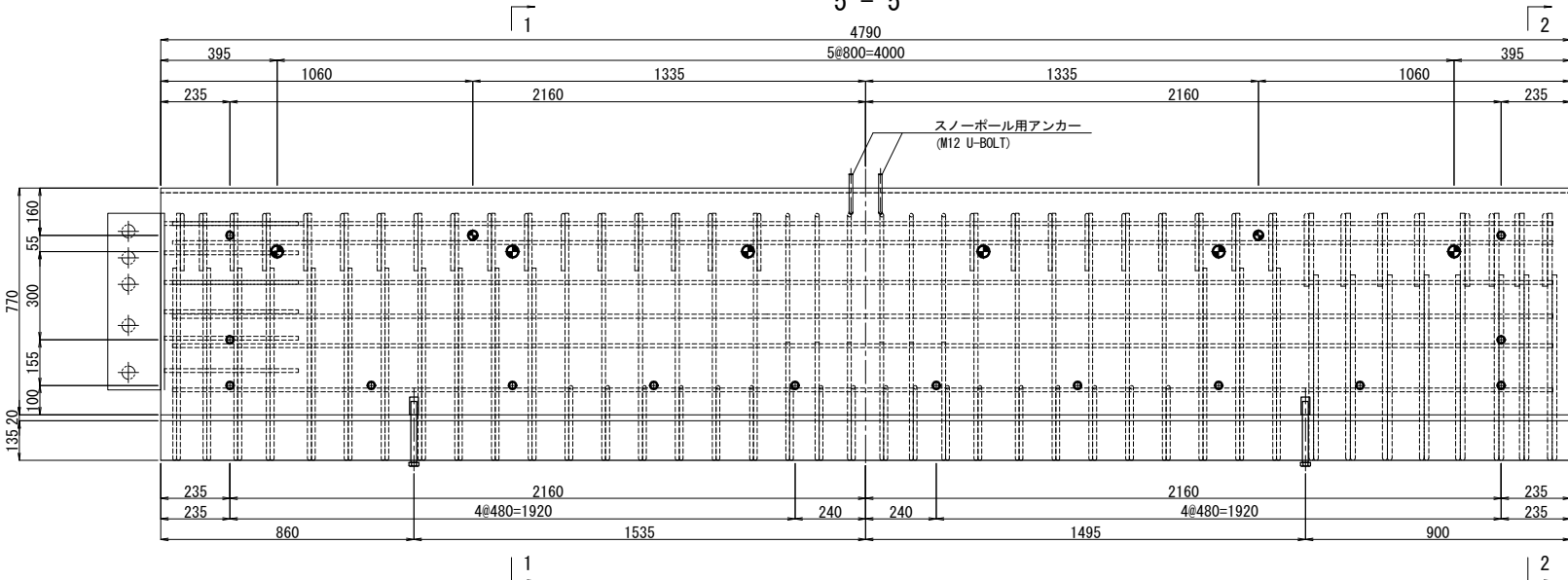
埋設管配置側面図
