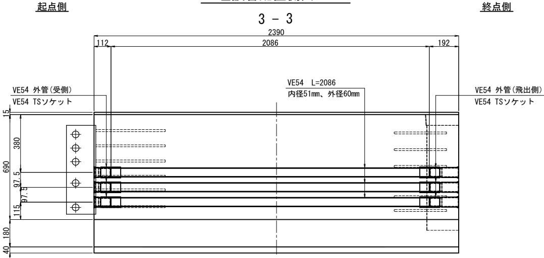
埋設管配置側面図
