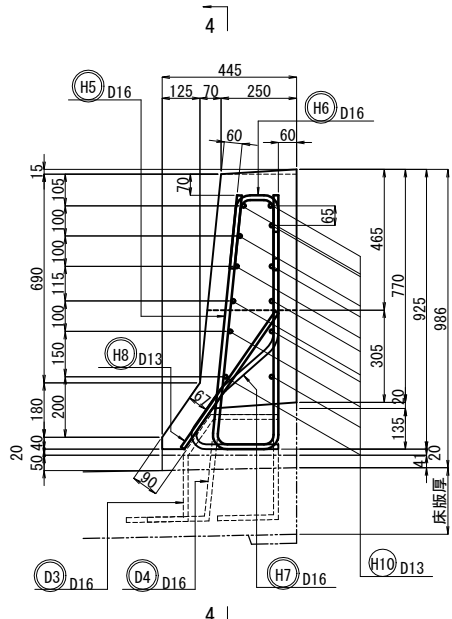
断面図
