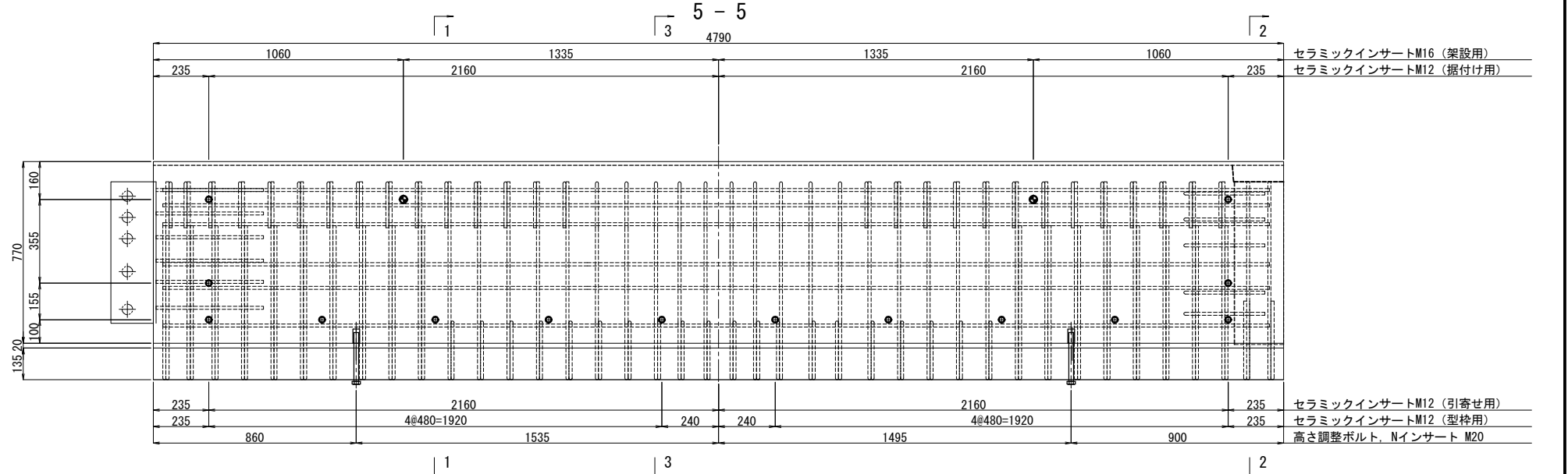
埋設管配置側面図
