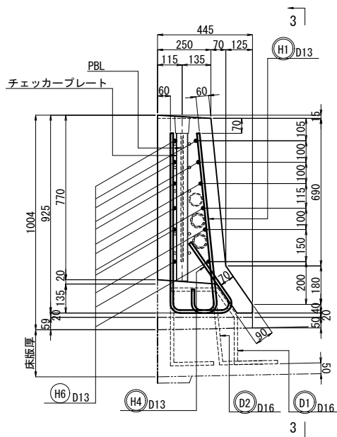
断面図 2 - 2
