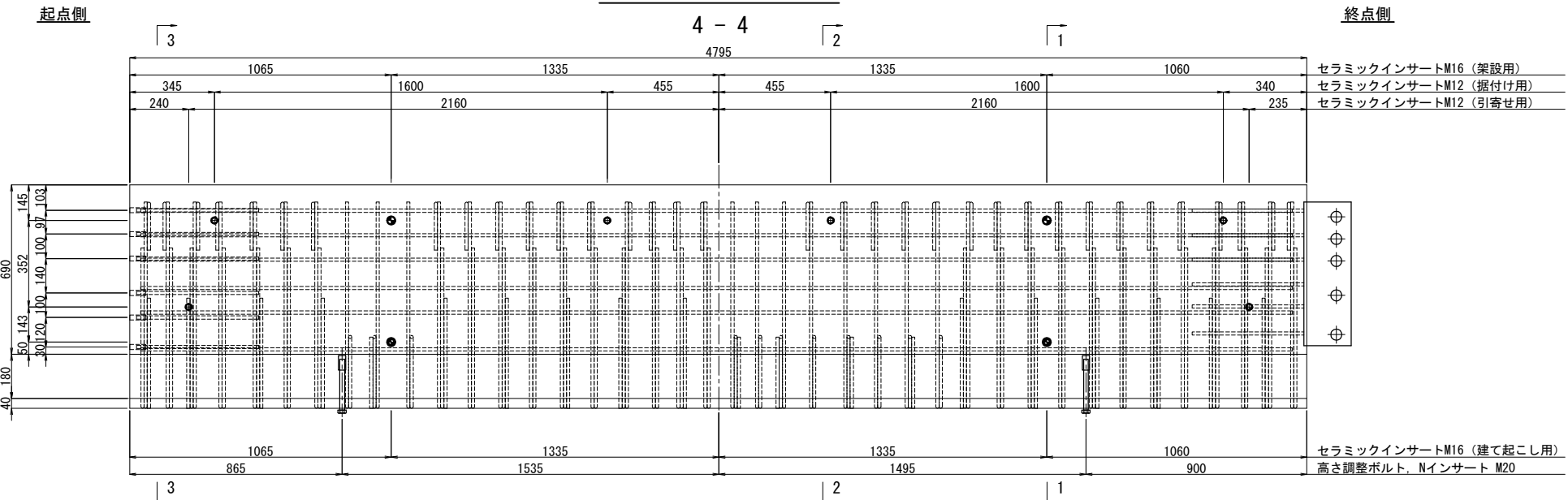
インサート配置側面図
