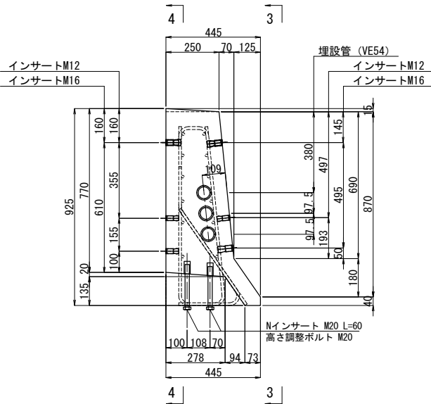
断面図 1 - 1
