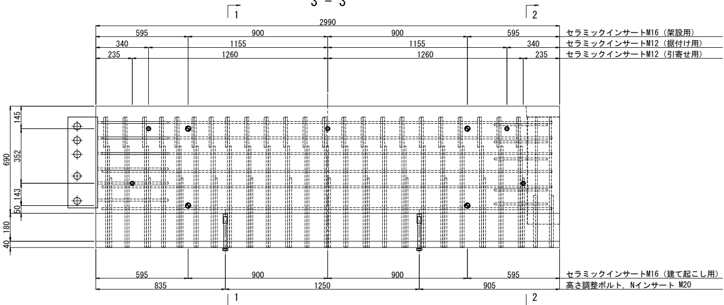
インサート配置側面図
