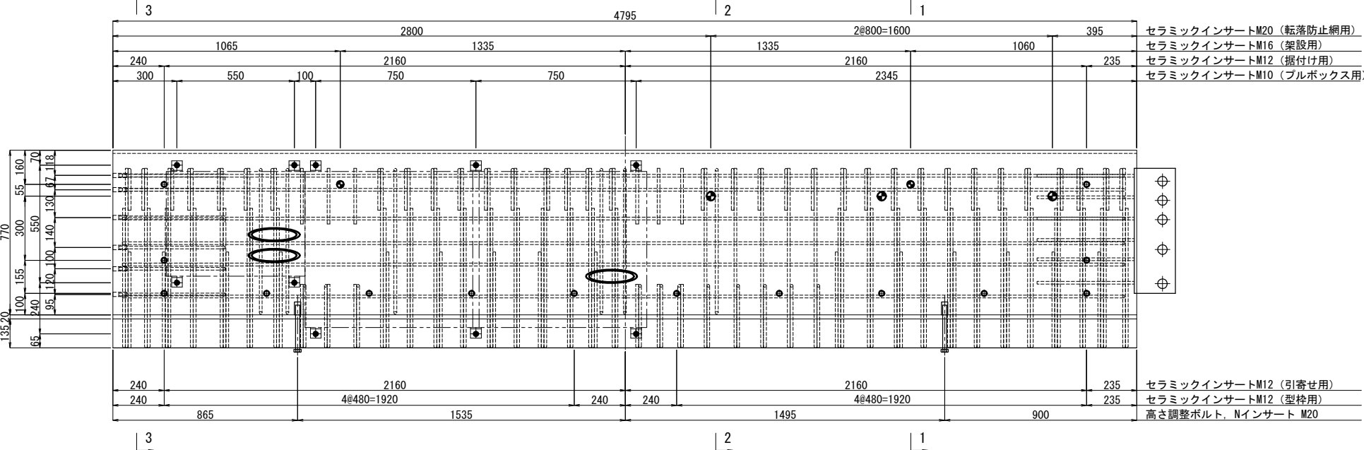
埋設管配置側面図
