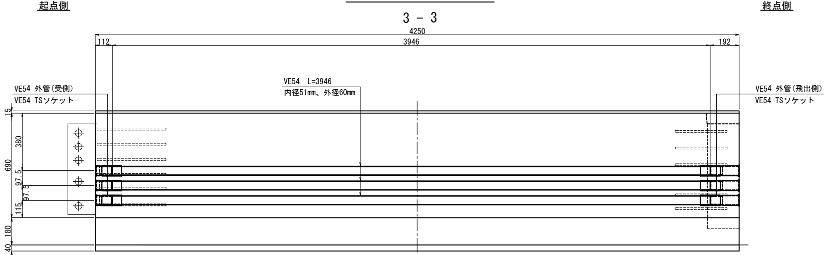
埋設管配置側面図
