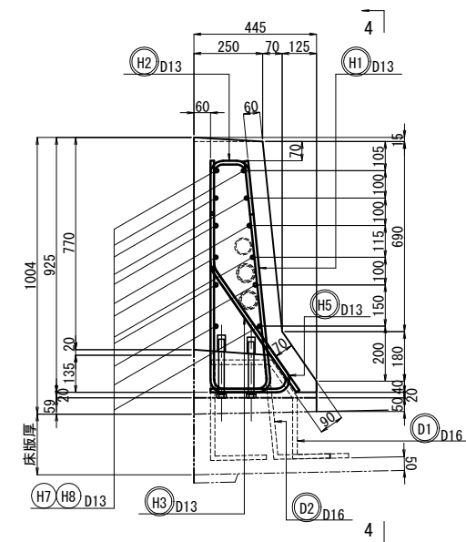
断面図 2 - 2
