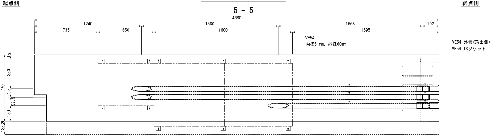
埋設管配置側面図
