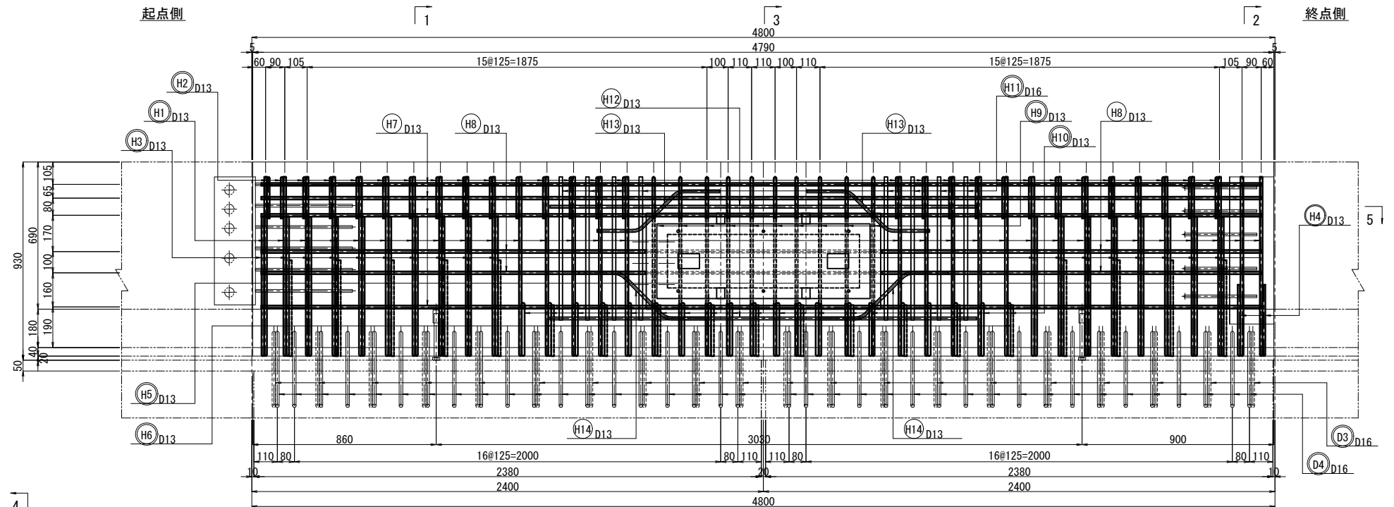
側面図 4 - 4
