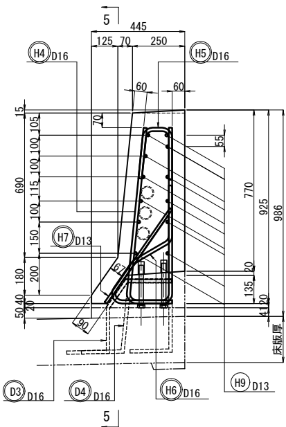
断面図
