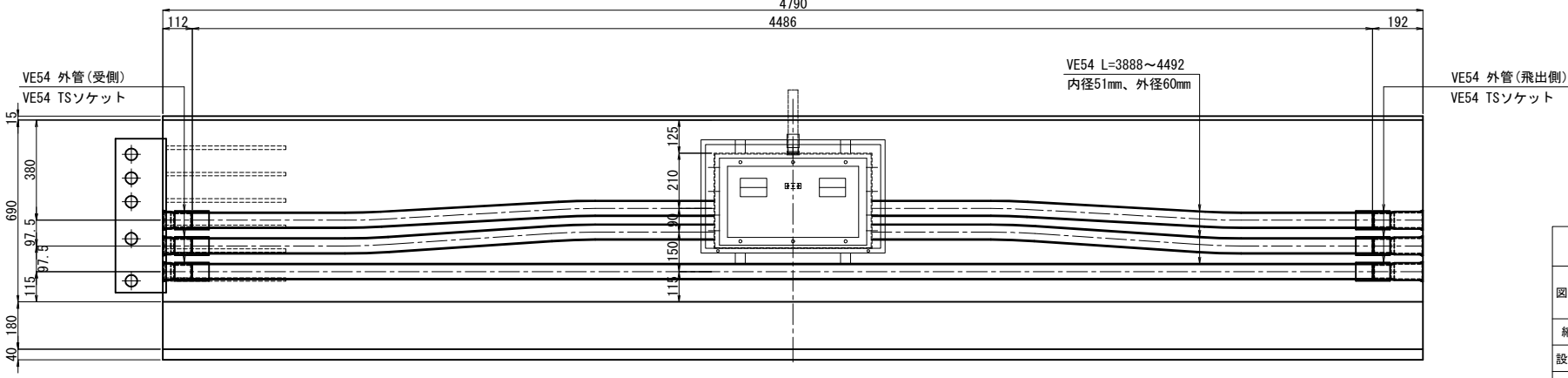
埋設管配置側面図
