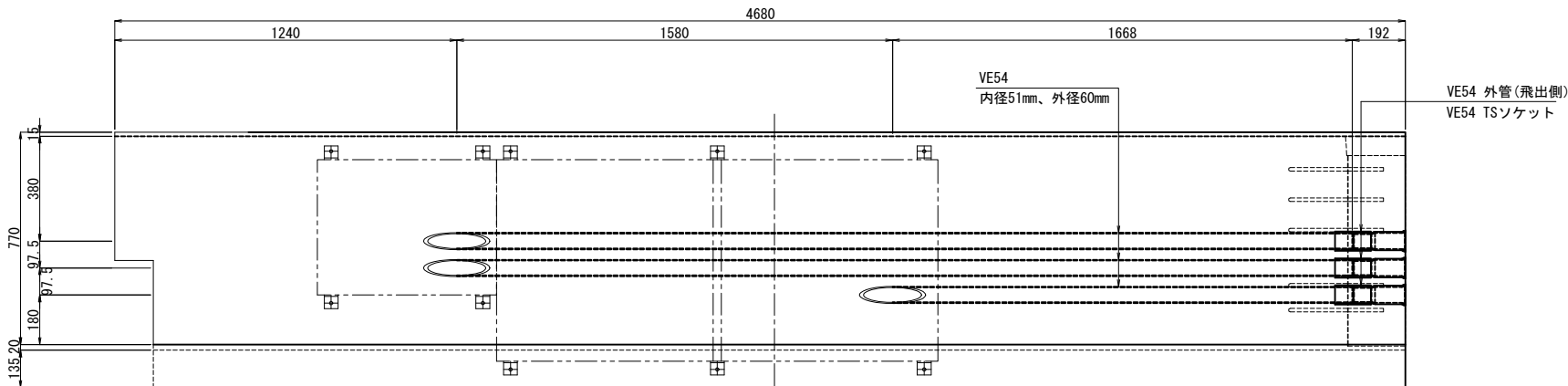
埋設管配置側面図
