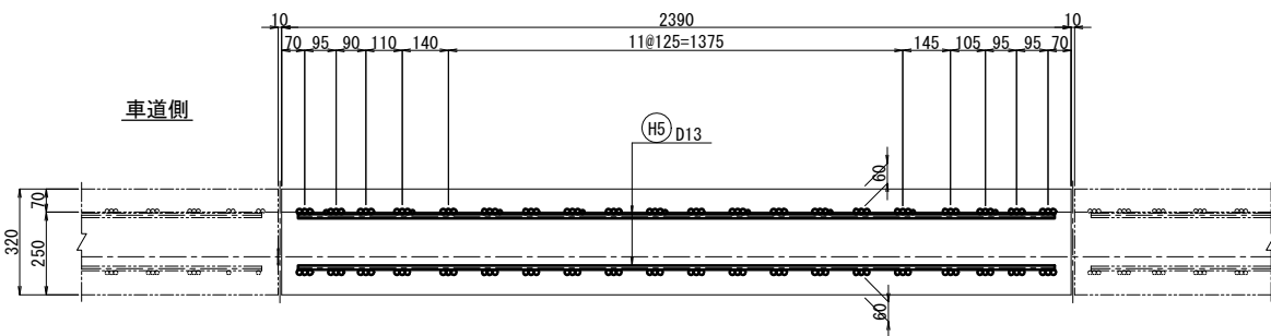
平面図
