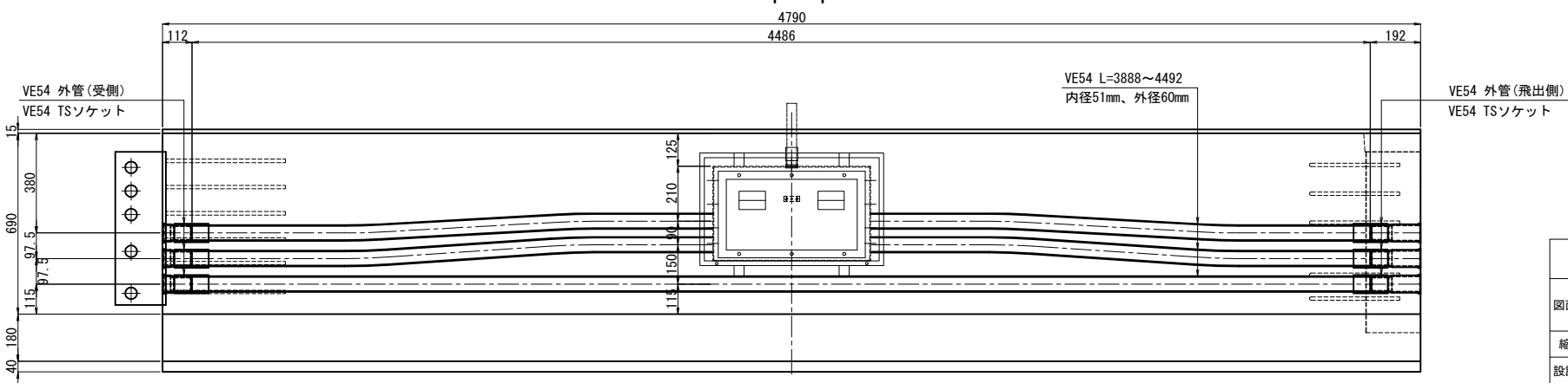
埋設管配置側面図
