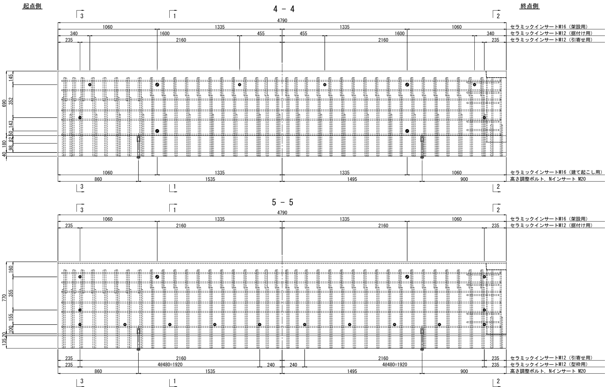
埋設管配置側面図
