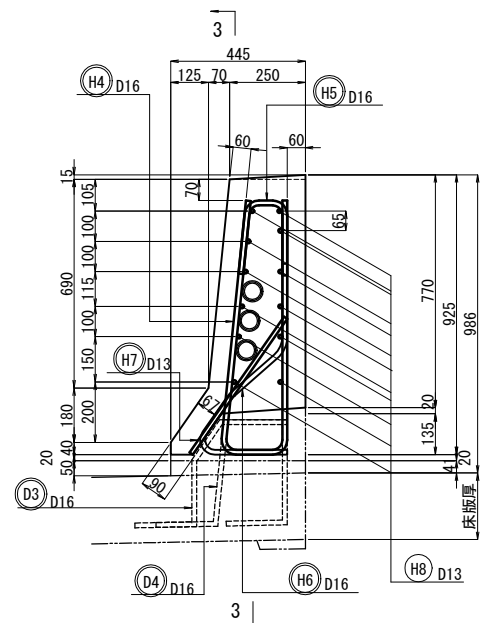
断面図
