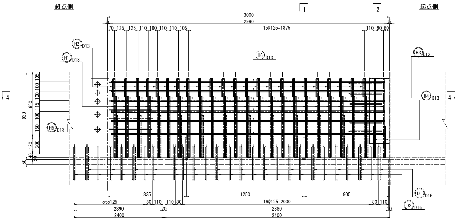
側面図
