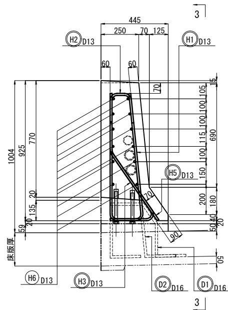
断面図 2 - 2
