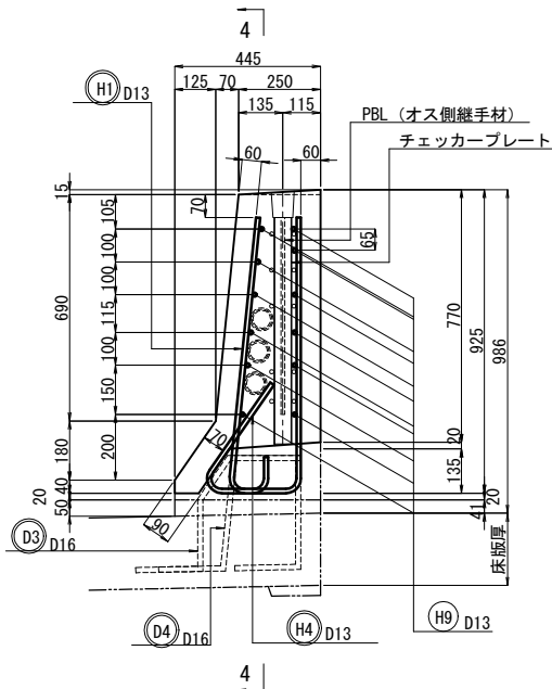
断面図
