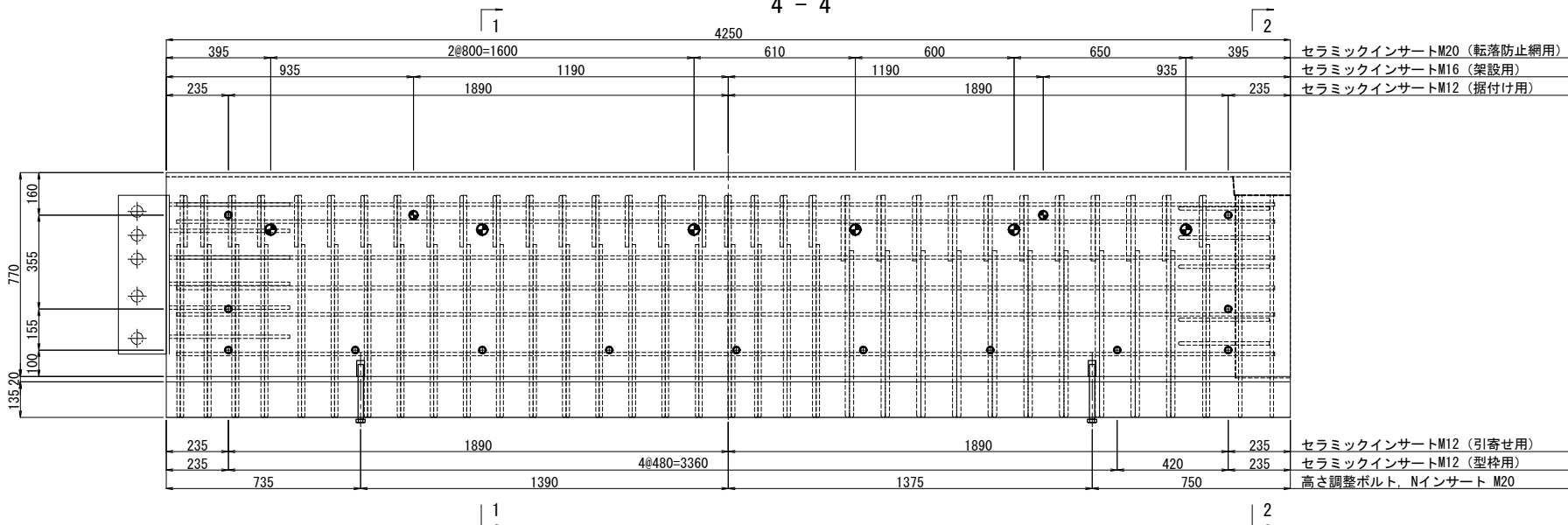
埋設管配置側面図
