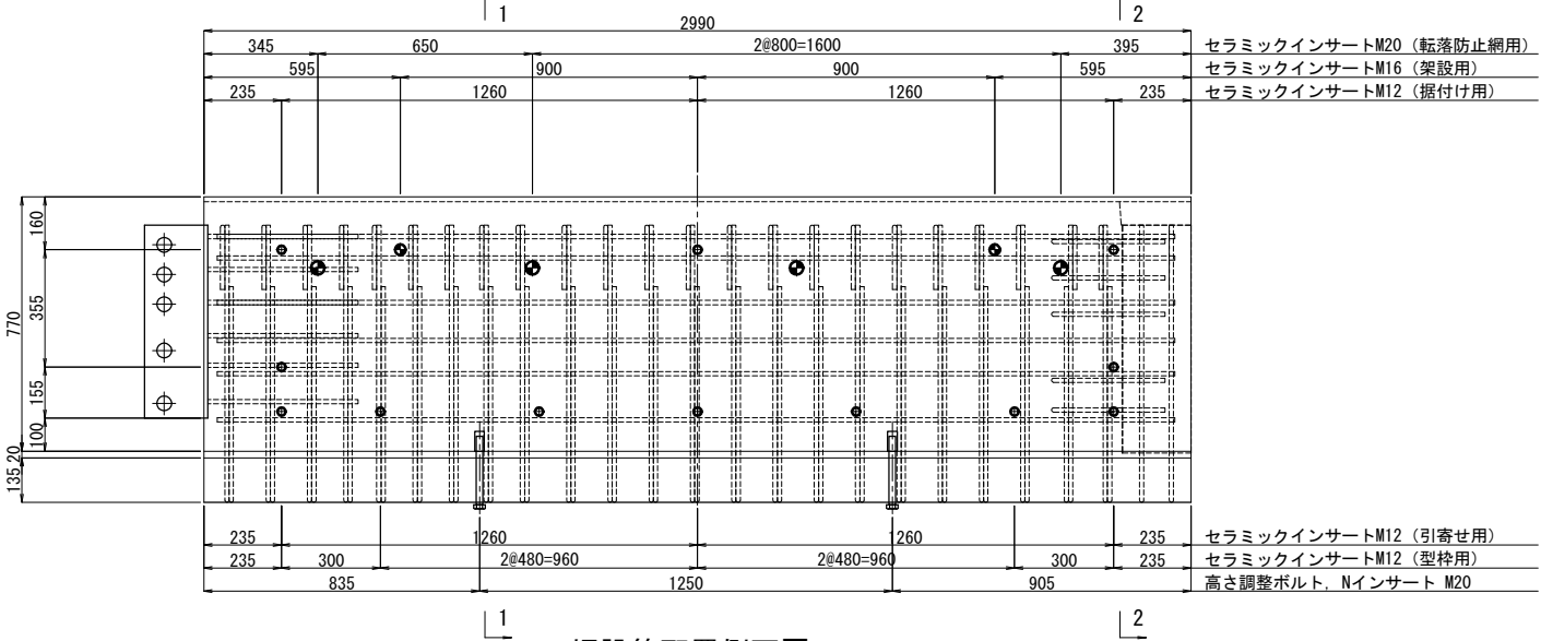
埋設管配置側面図
