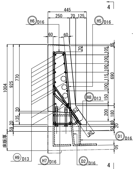
断面図 2 - 2
