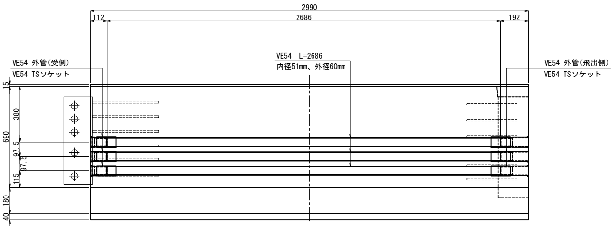
埋設管配置側面図
