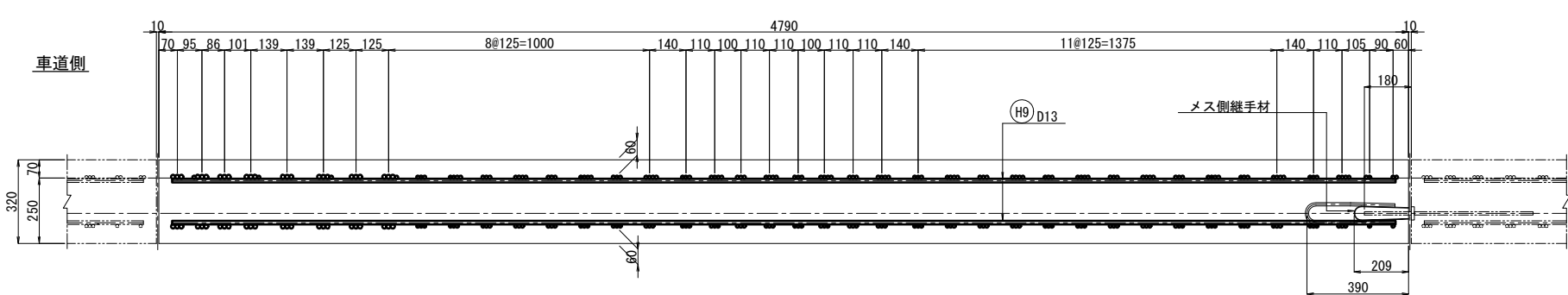
平面図
