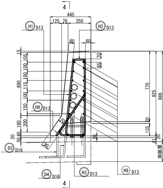
断面図
