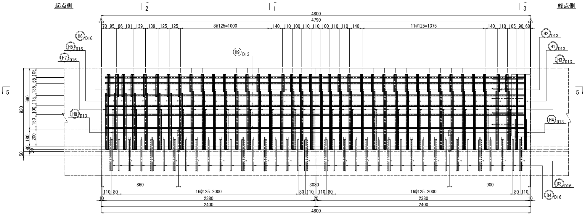
側面図
