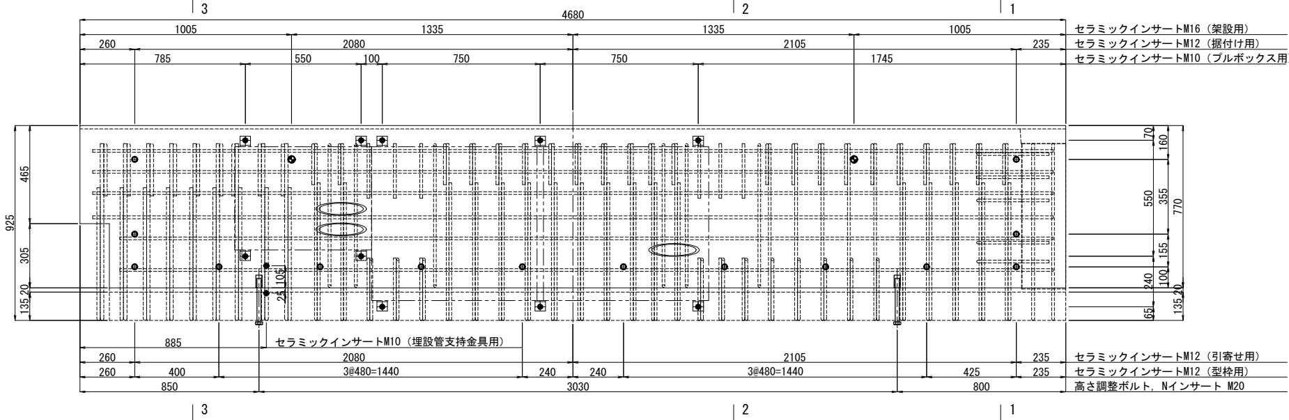
埋設管配置側面図
