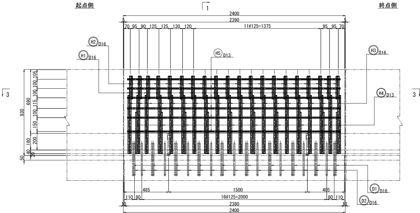
側面図
