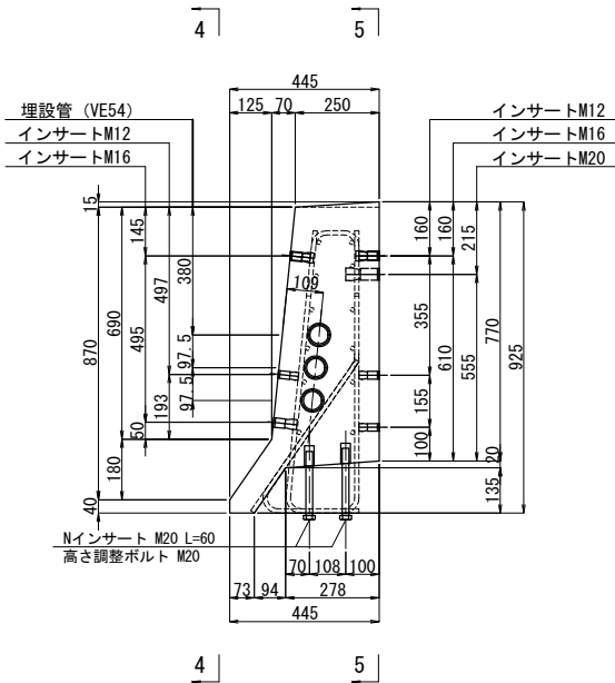
断面図 1 - 1
