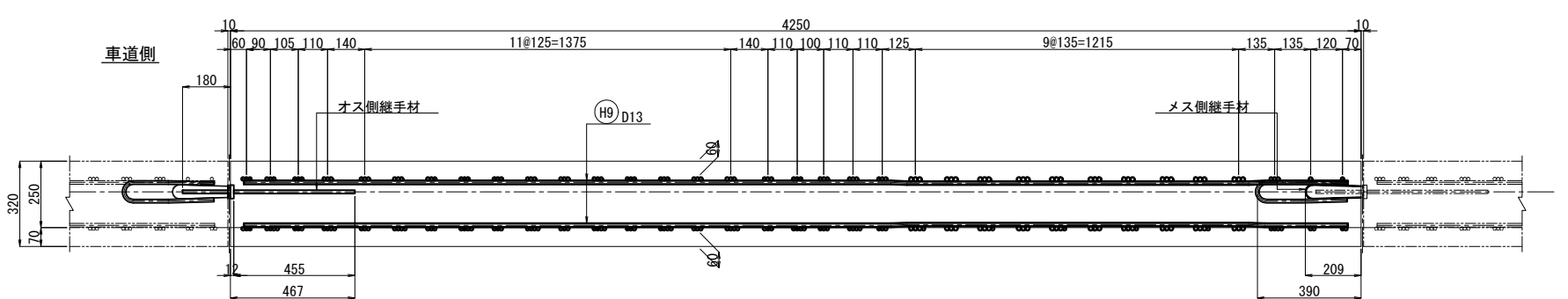
平面図
