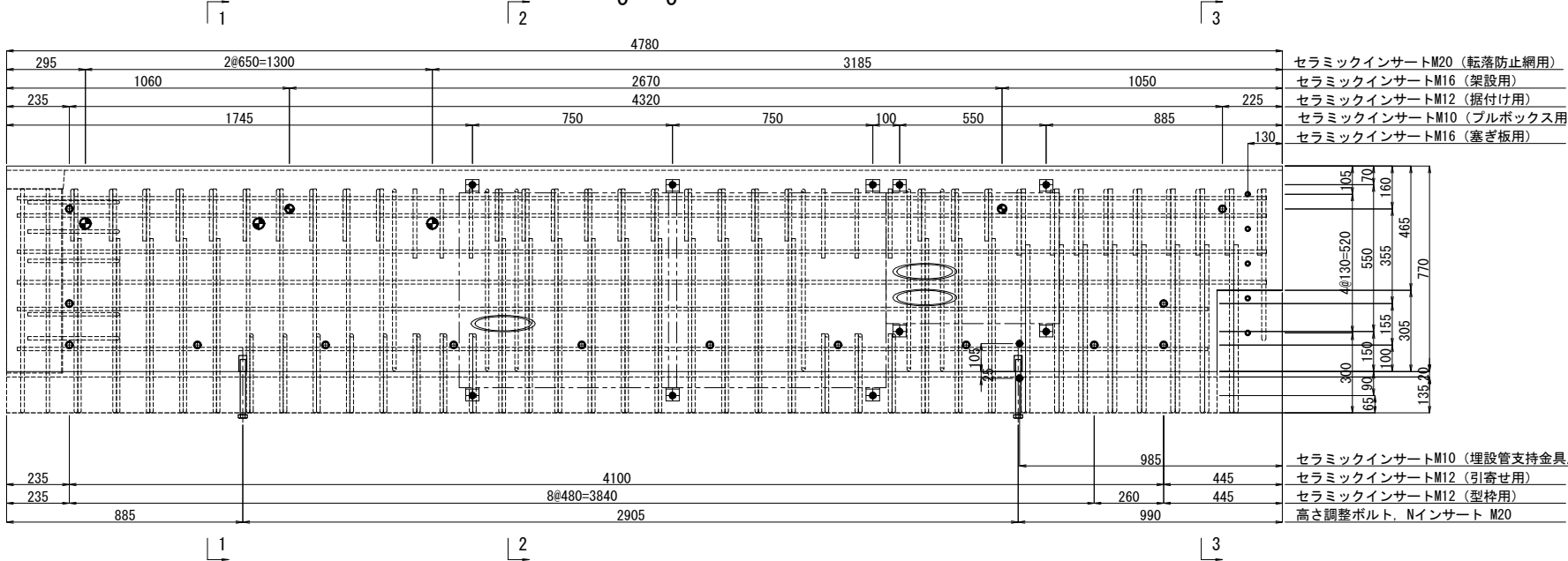
埋設管配置側面図
