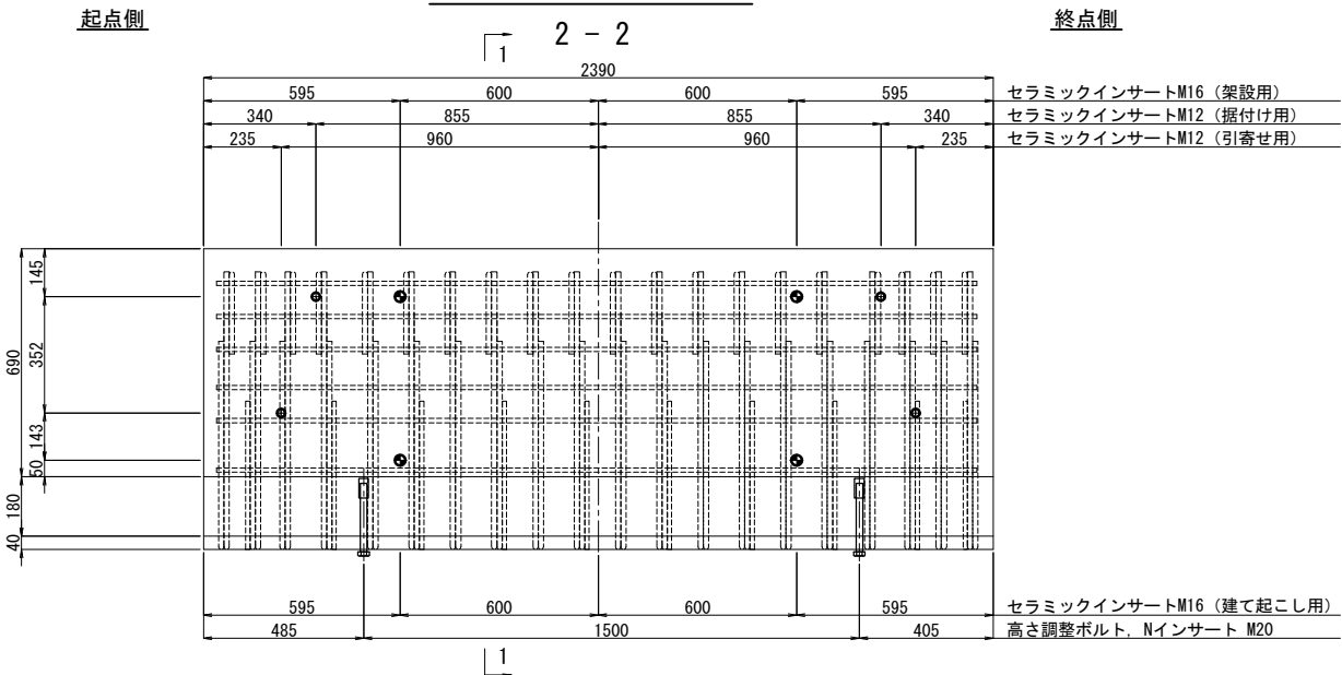
インサート配置側面図
