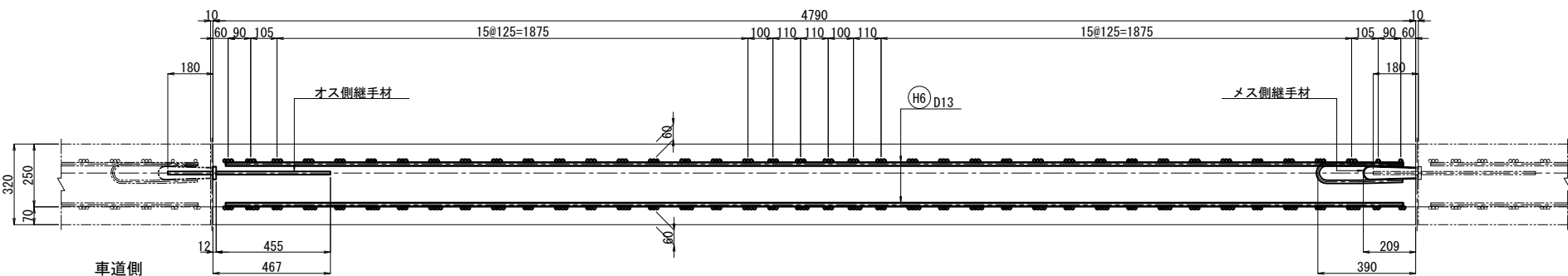
平面図 4 - 4
