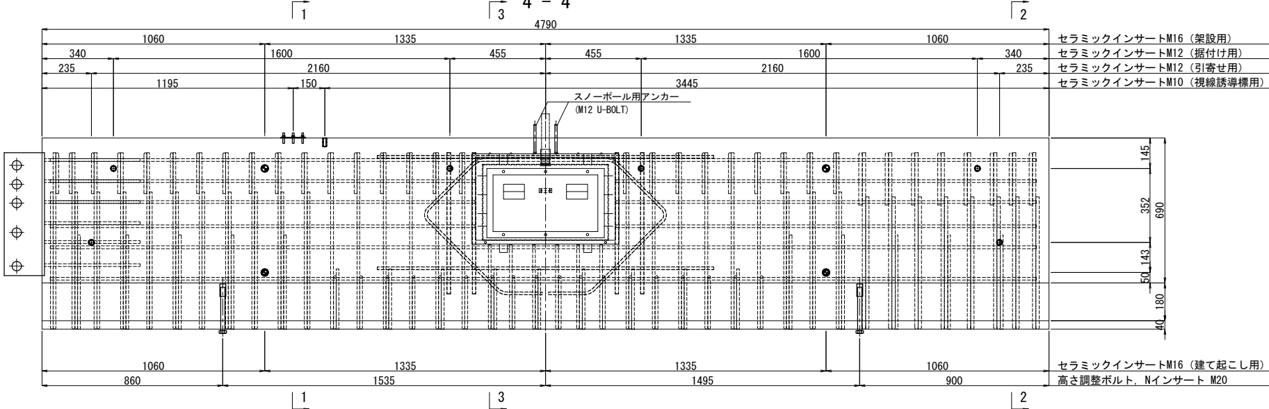
インサート配置側面図
