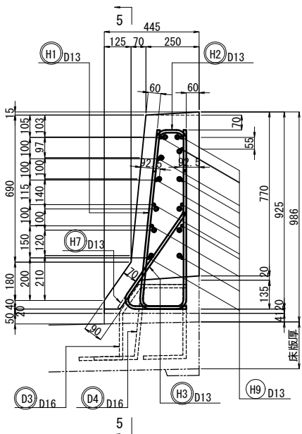
断面図
