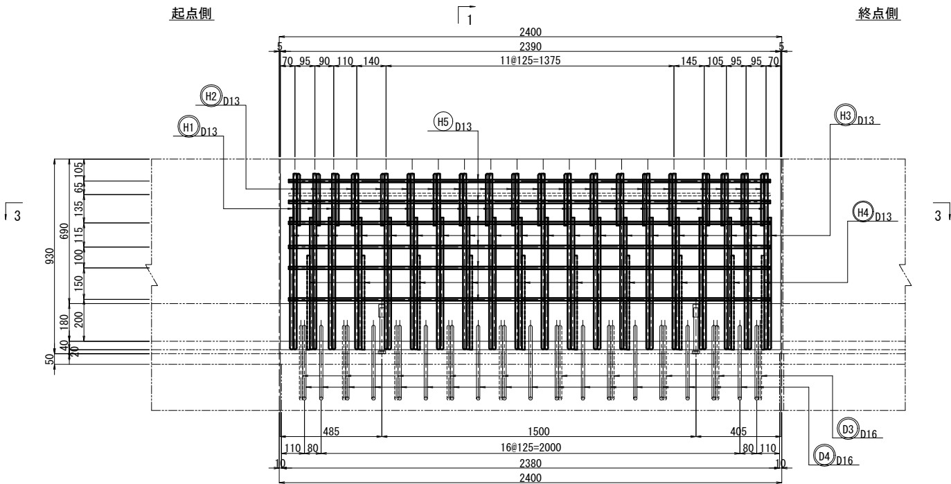
側面図
