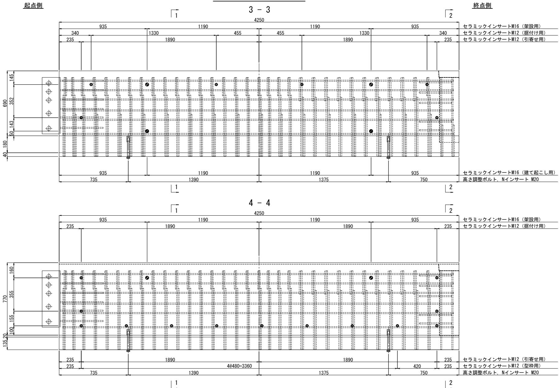
埋設管配置側面図
