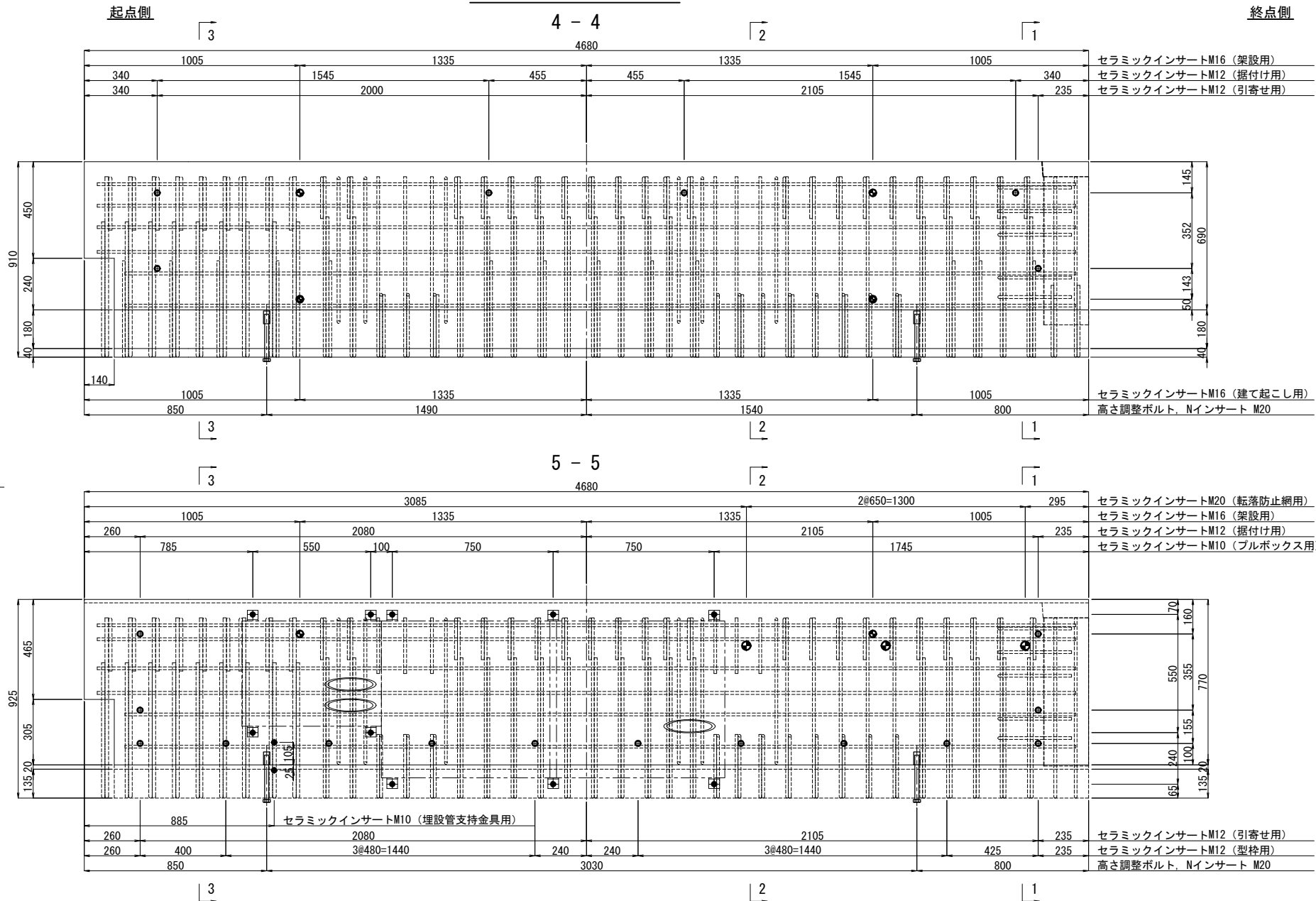
インサート配置側面図
