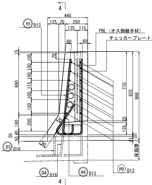
断面図
