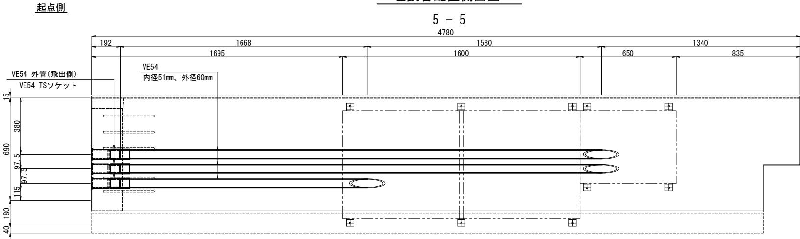
埋設管配置側面図
