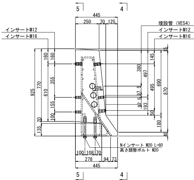
断面図
