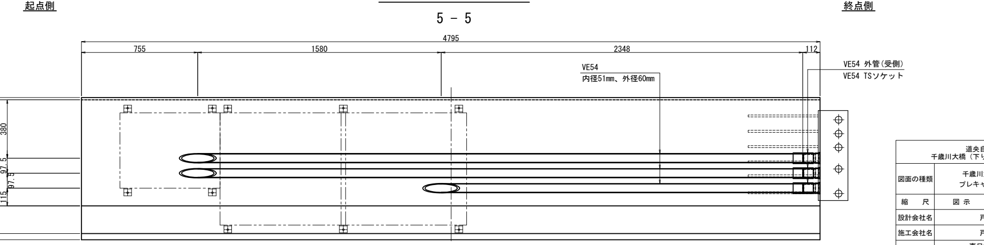
埋設管配置側面図
