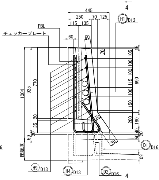
断面図 3 - 3
