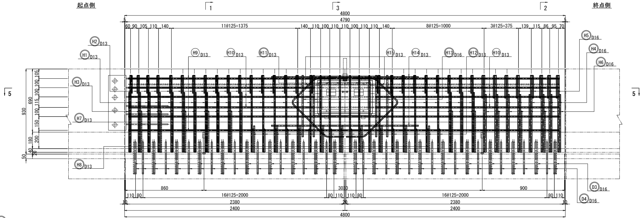
側面図
