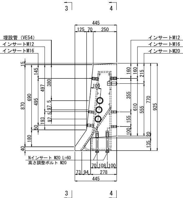
断面図 1 - 1
